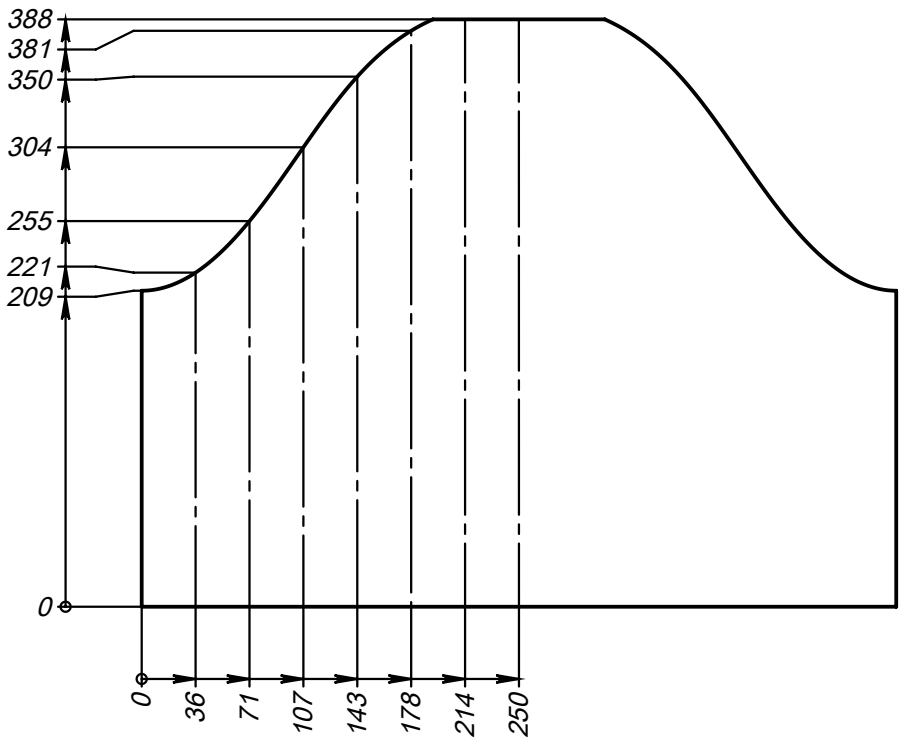
Поз.2 (Труба) развертка
